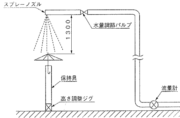
<人工降雨試験装置>
